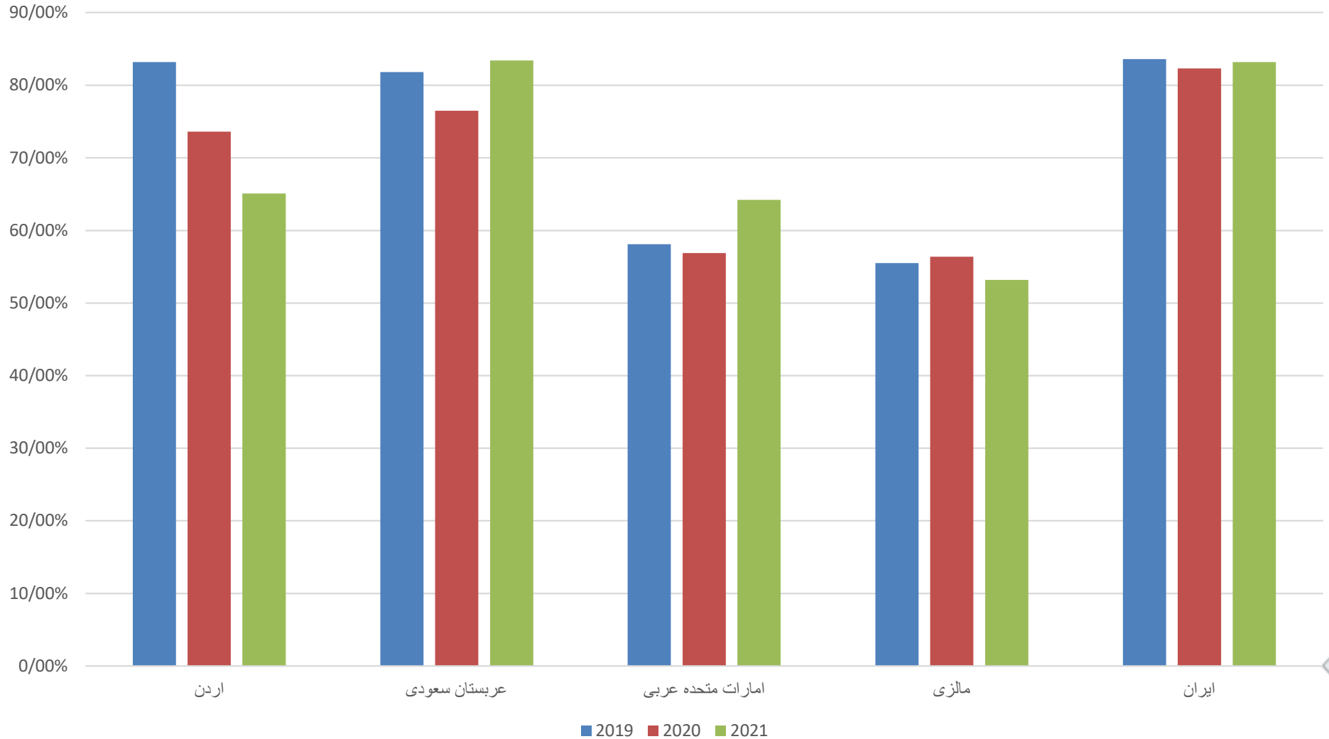
ضریب خسارت
